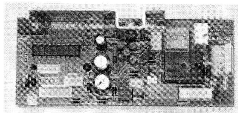
Power PCB KW715253
